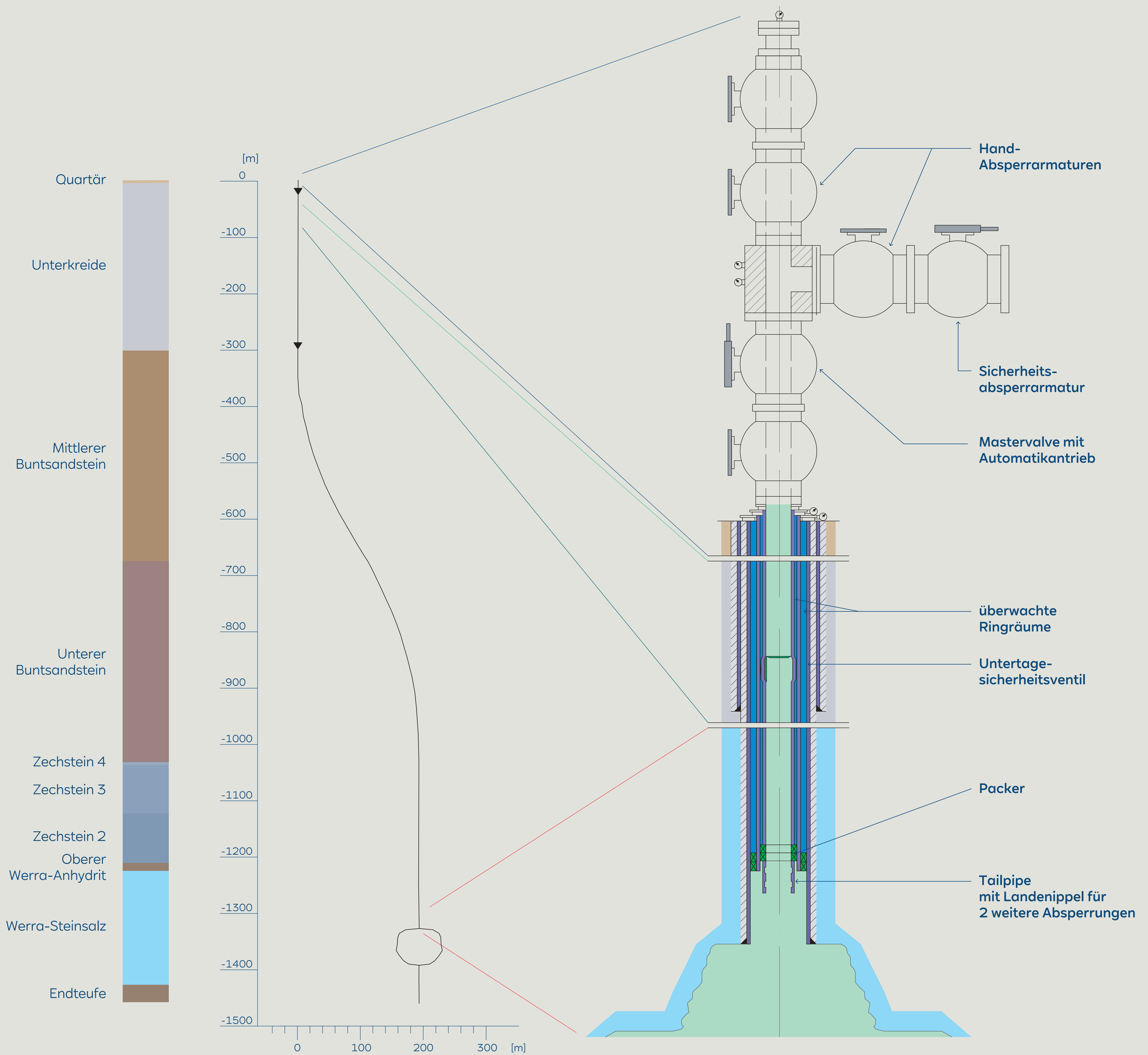
Maßstäbliche Darstellung
